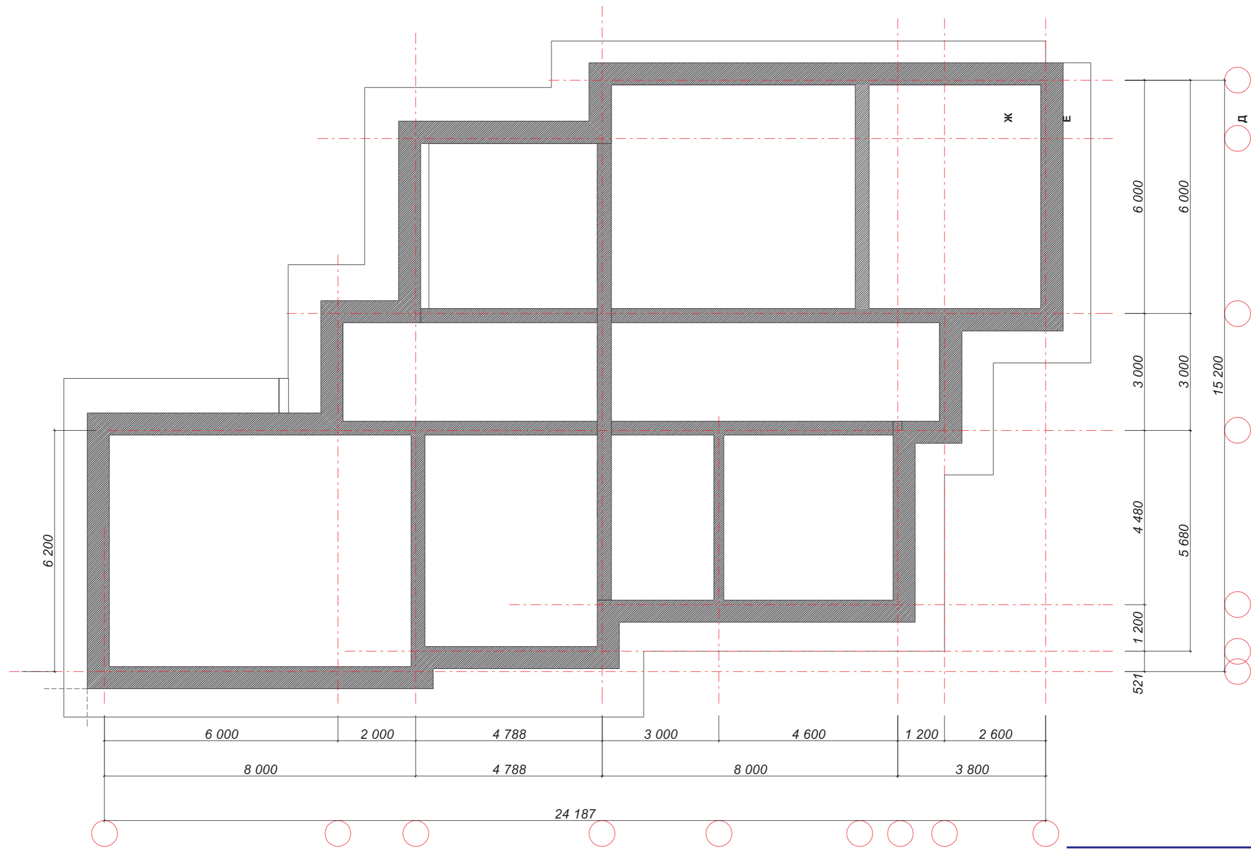
план фундамента М 1:100
