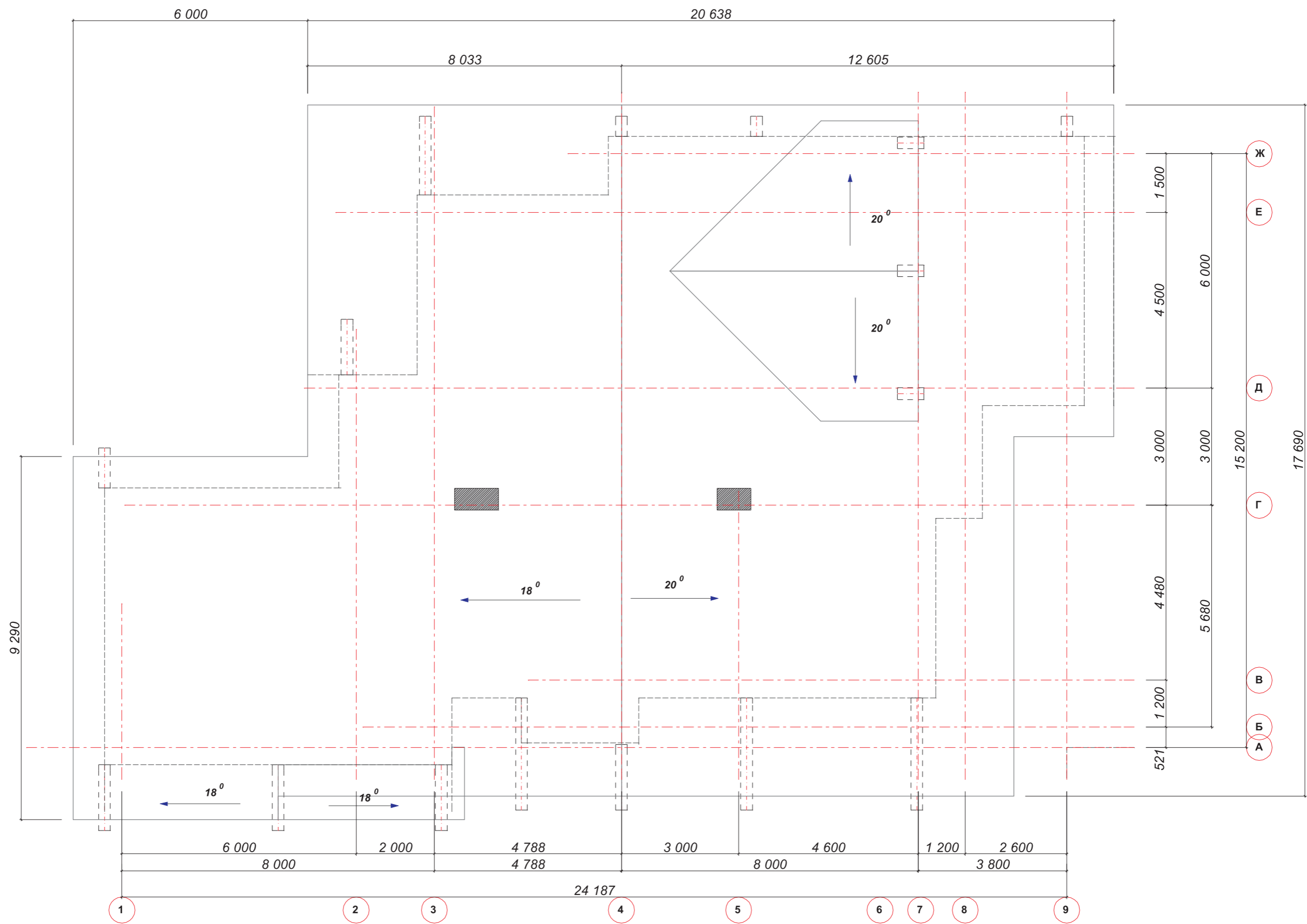
план кровли М 1:100
