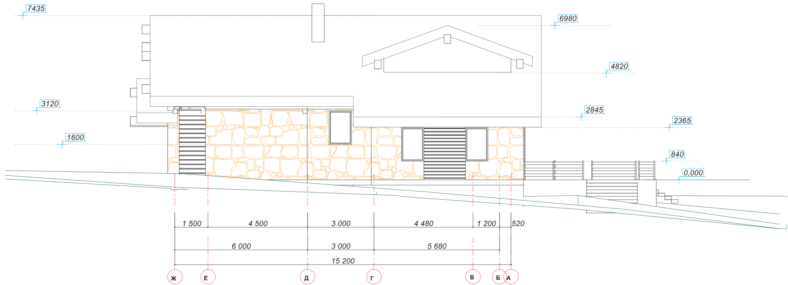
фасад в осях А-Ж, Ж-А М 1:100
