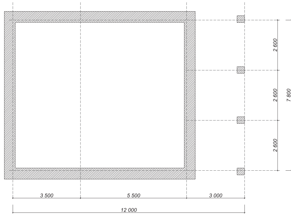
план фундамента М 1:100
